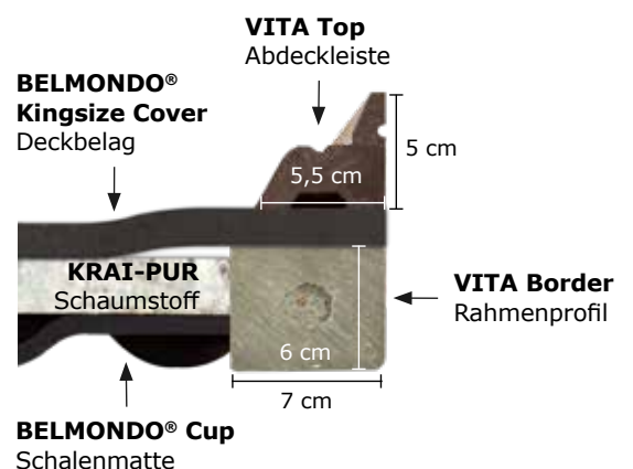
bewährtes Hammer-schlagprofil
